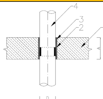
Rys. 2. Przejście w stropie
