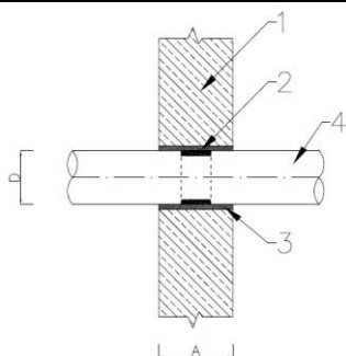
Rys. 1. Przejście w ścianie
