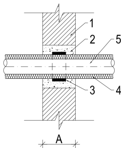
Rys. 7. Pojedyncza rura niepalna z kauczukiem w ścianie
